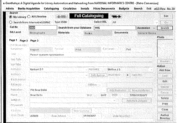
figure-2: Cataloguing Module
